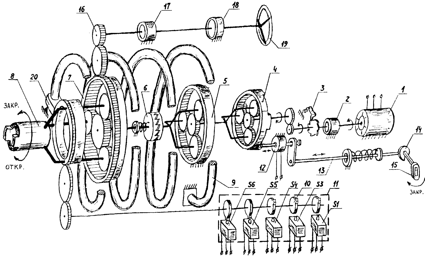
ПРИЛОЖЕНИЕ Б Кинематическая схема механизма МБОВ-63/1-0,25(У)
