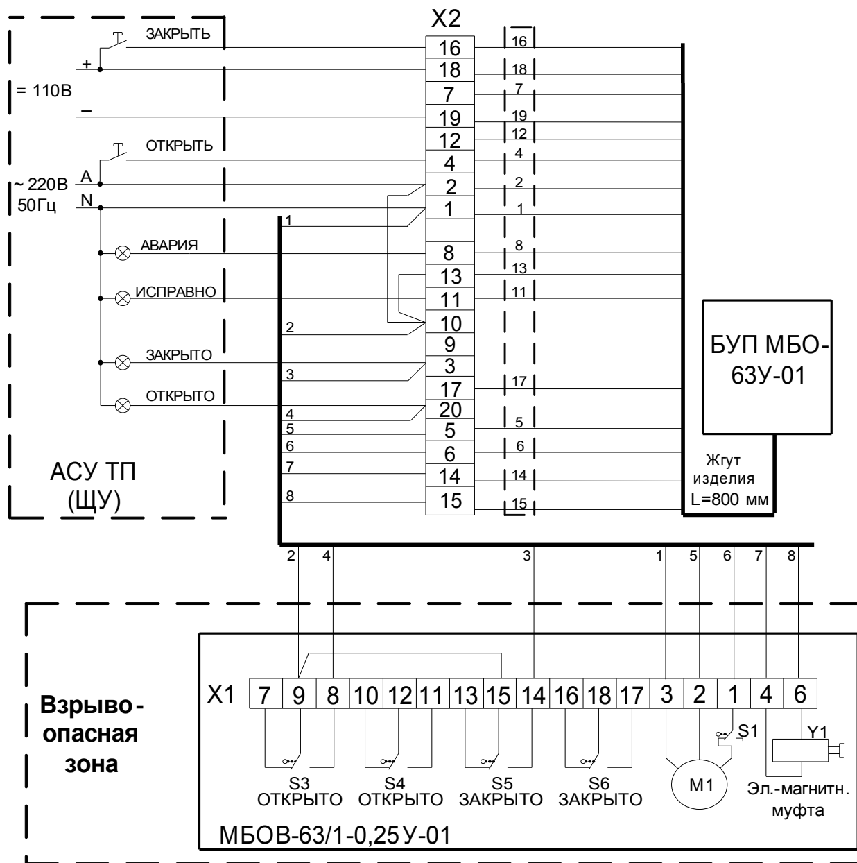
Схема электрическая подключений электромеханизма МБОВ -63/1-0,25У-01 с блоком БУП МБО-63У-01
